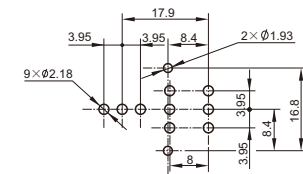
70A、80A、100A PCBtype
