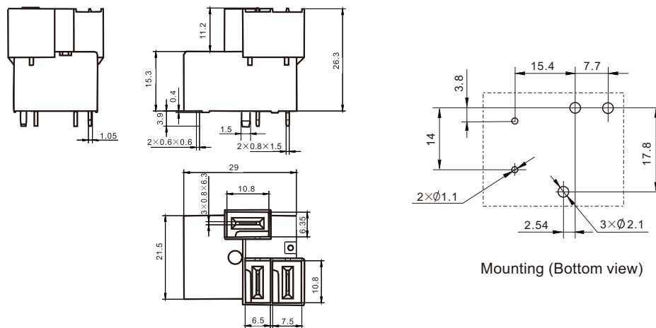
Dimensions
