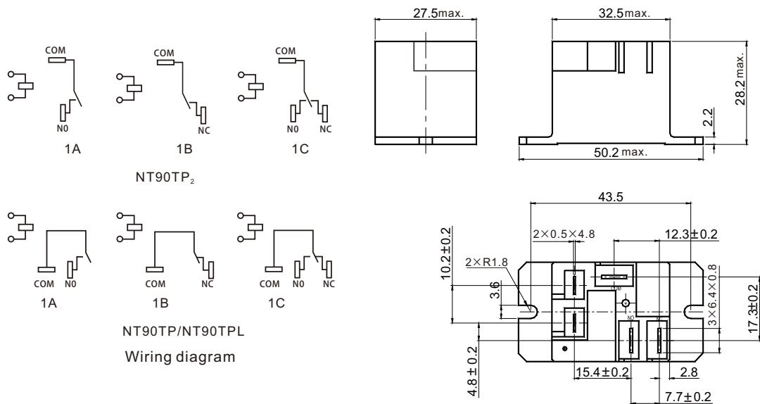
NT90TP 2 Dimensions
