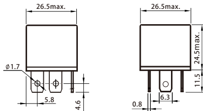
NVF4-1type
