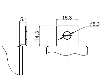
NVF4-1type
