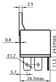
NVF4-2 type
