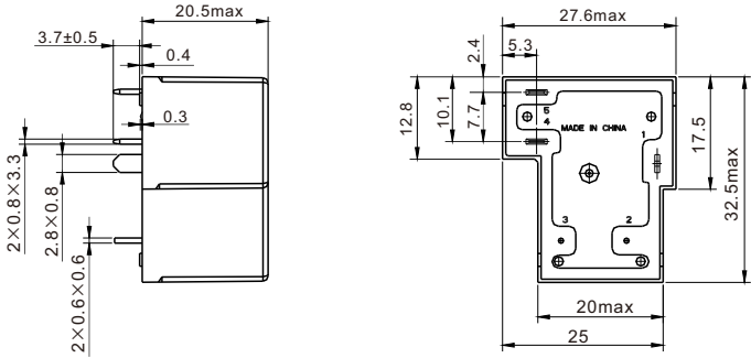
Dimensions
