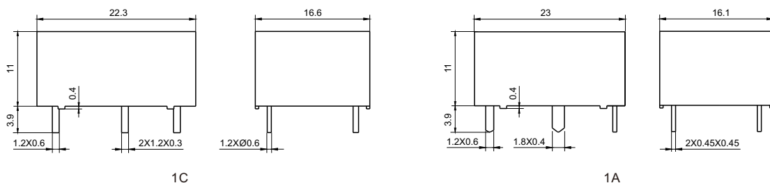
Dimensions
