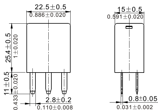
外形尺寸图
