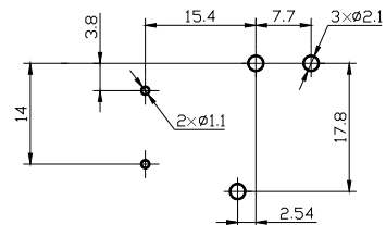
安装尺寸图 (底视图)
