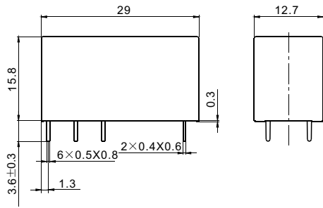
外形尺寸图
