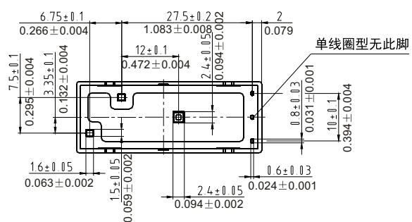
安装尺寸图 (底视图)
